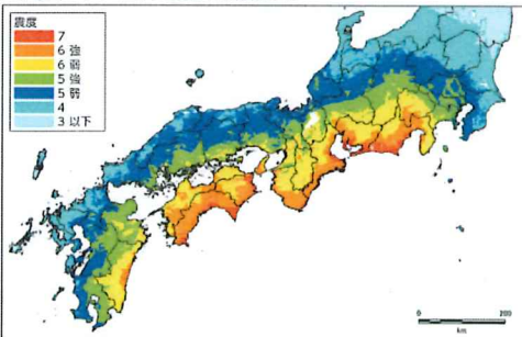
■ 南海トラフ巨大地震の震度分布
